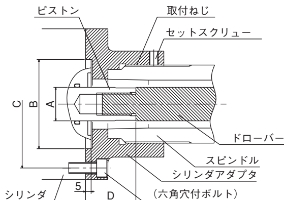
図9 シリンダアダプタ取付部
