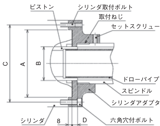
図10 シリンダアダプタ取付部
