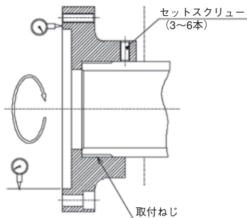
図11 シリンダアダプタの振れ測定
