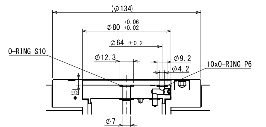
テーブル面詳細 DETAIL OF TABLE
