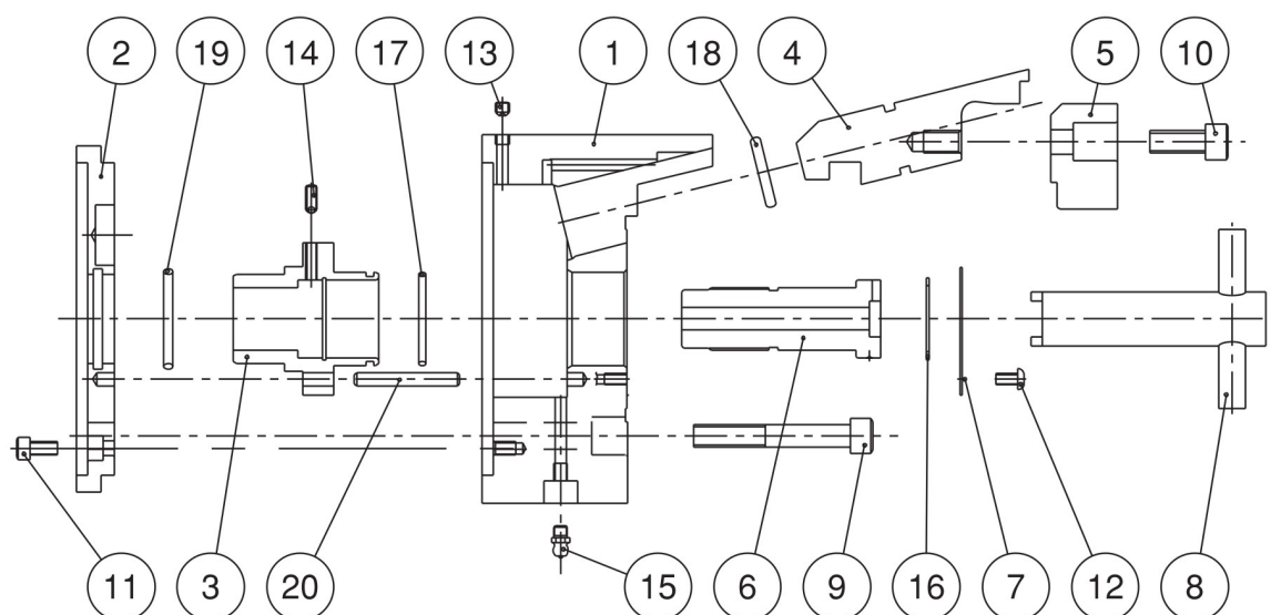
図 5 PU206～PU212形
