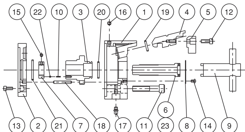
図 4 PU203～PU205形
