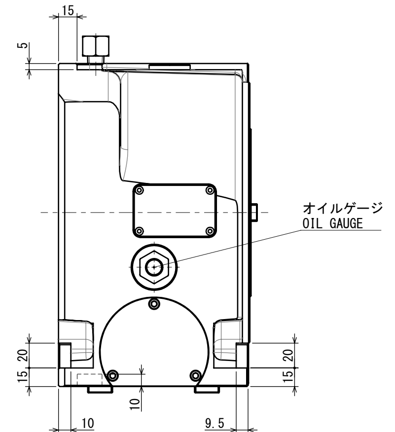
A矢視／VIEW A
