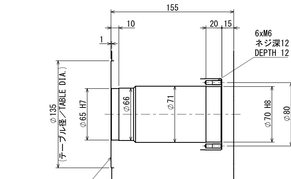
スピンドル穴／SPINDLE THRU-HOLE
