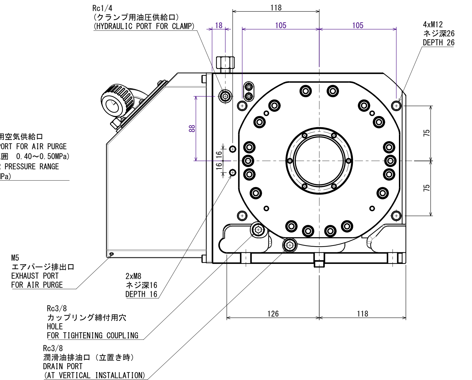
A矢視／VIEW A
